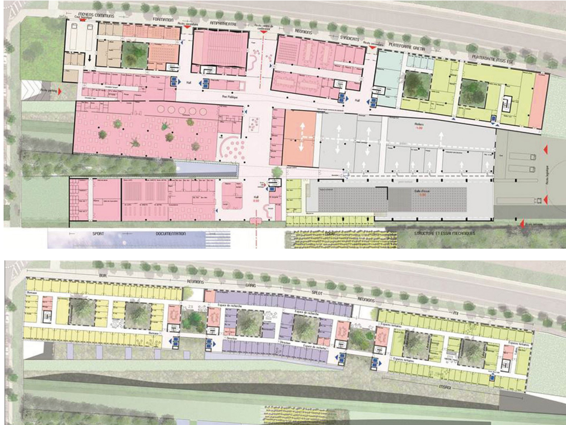
REALISATION DE L'ESPACE BIENVENUE, POLE SCIENTIFIQUE ET TECHNIQUE
